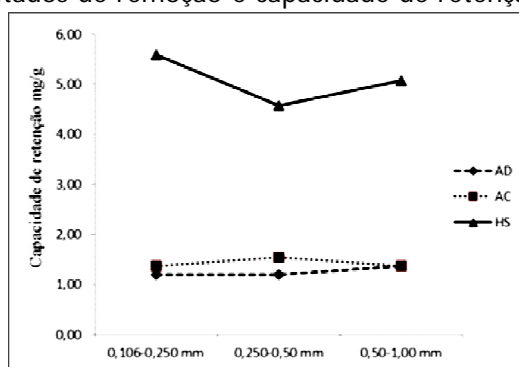
Figura 1: Capacidade de retenção versus tamanho de partículas. As diferentes linhas são referentes aos tratamentos químicos: AD, água deionizada; AC, ácido clorídrico; HS, hidróxido de sódio.
