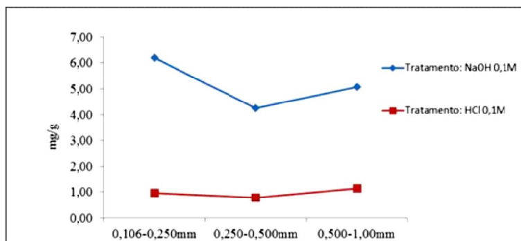
Figura 1: Adsorção de Cálcio(II) em cada material adsorvente obtido.
