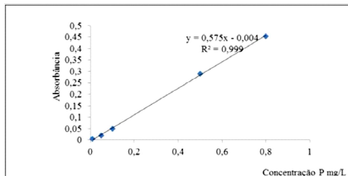
Figura1. Curva de calibração por padrão externo dos valores de absorbância versus concentração de fósforo (P).
